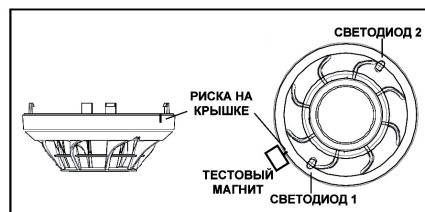
Рис. 3: Тестирование магнитом
